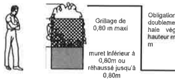
Cas 2 : muret existant inférieur à 0,80 mètre
